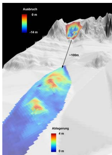
Abb.1: Quantifizierung eines Felssturzes aus dem Jahr 2008 im Val di Funes/Dolomiten (ermittelt aus einer Cut an Fill-Analyse)
